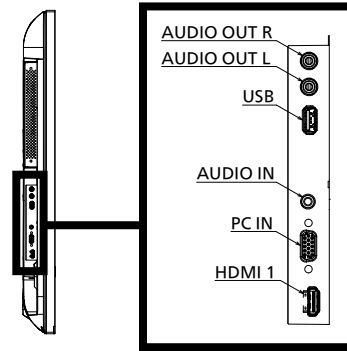
端子部拡大図a
