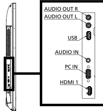
端子部拡大図 a
