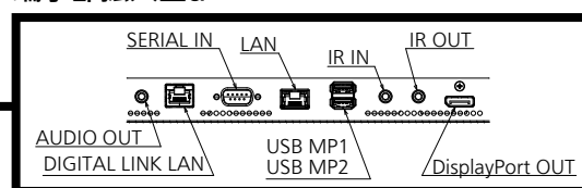
端子部拡大図 a
