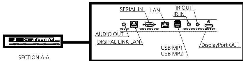
端子部拡大図 a
