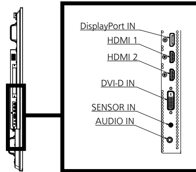
端子部拡大図 b
