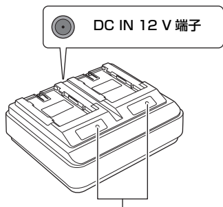
充電ランプ [CHARGE1/CHARGE2]
