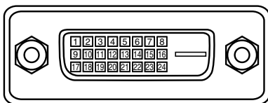
DVI-D 24ピン
