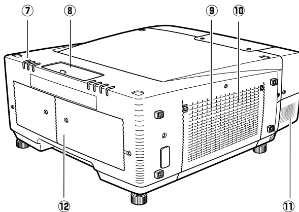
後面
