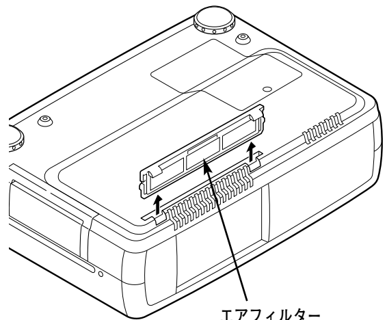
エアフィルター 両端のツメを上に取り上げて取り外します。
