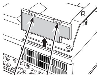
エアフィルター ツメを上を引き上げて 取り外します。
