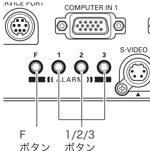
後面端子
