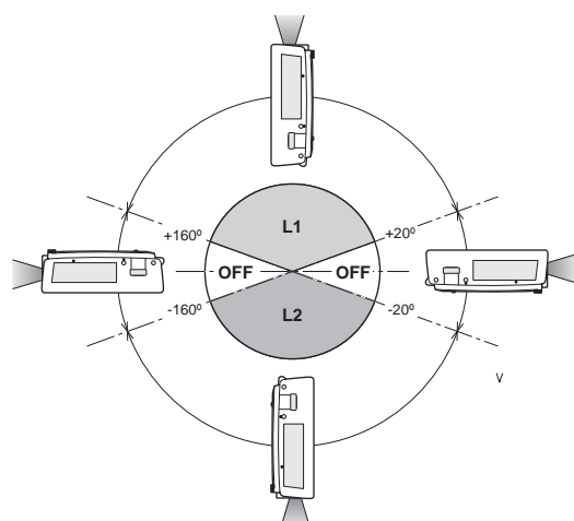
設置傾斜角度と「傾斜設定」の設定範囲
