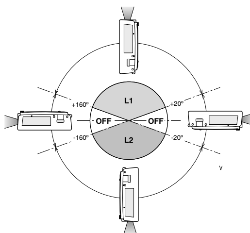
設置傾斜角度と「傾斜設定」の設定範囲
