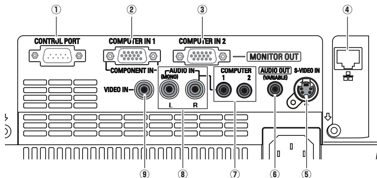
後面端子
