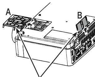
エアフィルター (A、B) 外側に引き出して取り外します。
