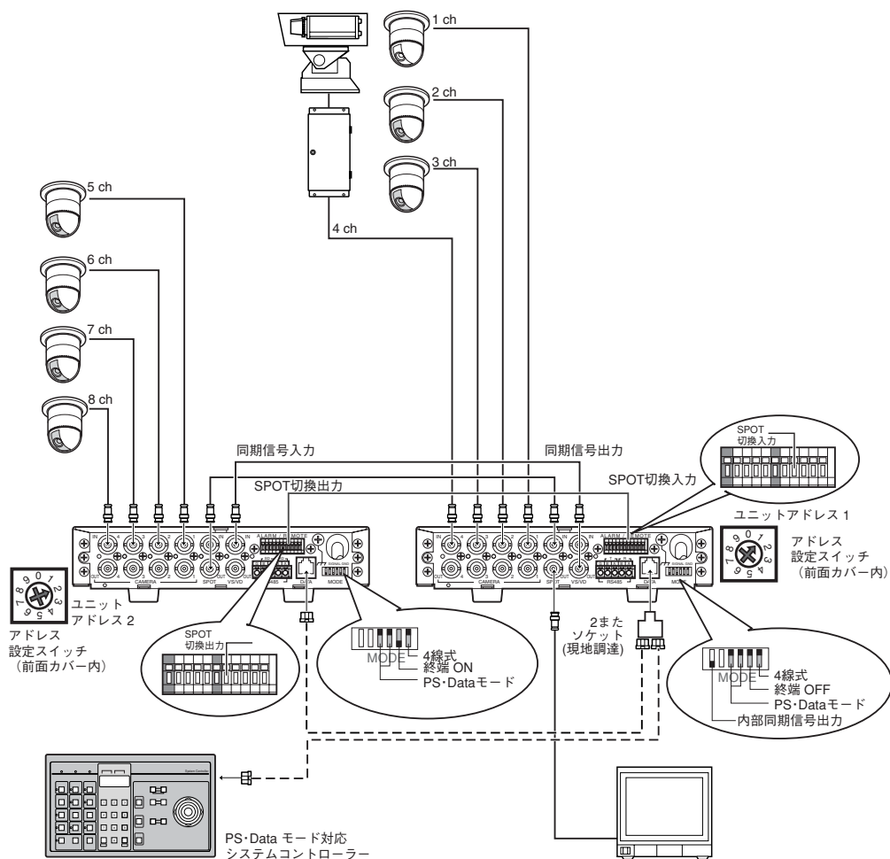
例2：本機を2台使用する場合のシステム例
