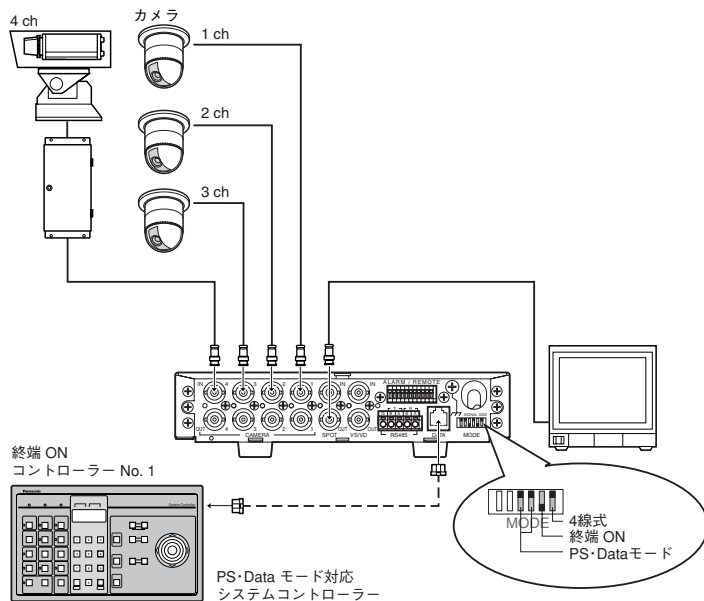
例1：本機を1台使用する場合のシステム例
