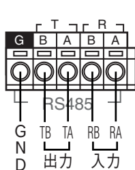
[本機後面から見た図]
