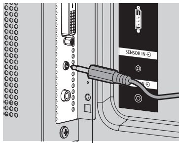
4 極超ミニケーブル
